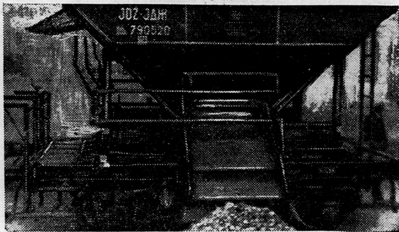
Naš prvi domači vagon za avtomatično razkladanje na odprti progi.
