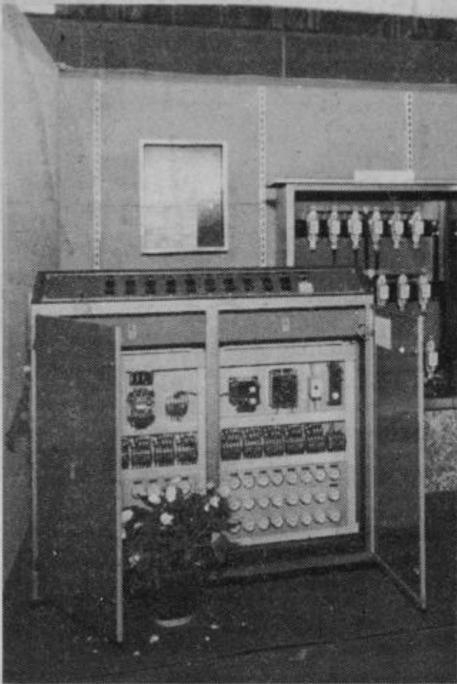
Elektro stikalna naprava pri sušilnici usnja
