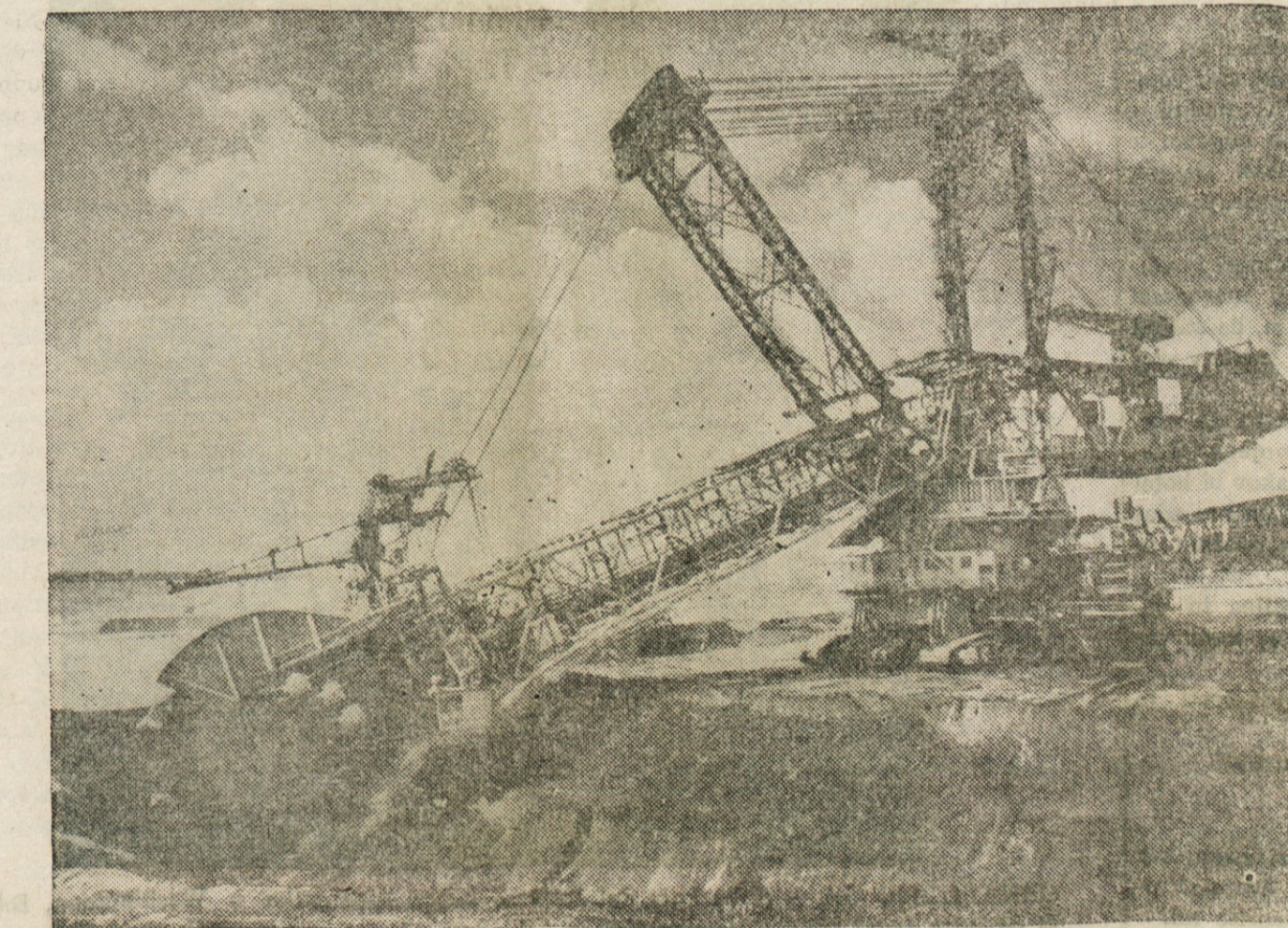
ORJAK SVOJE VRSTE — Slika kaže orjaški bager za kopanje premoga, ki so ga izdelali v Zahodni Nem-čiji. Sposoben je v 20 urah nakopati do 110,000 ton premoga.
