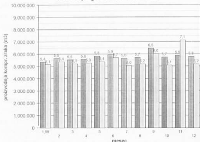
Proizvodnja komprimiranega zraka – mesečni pregled za leto 1998 in 1999
