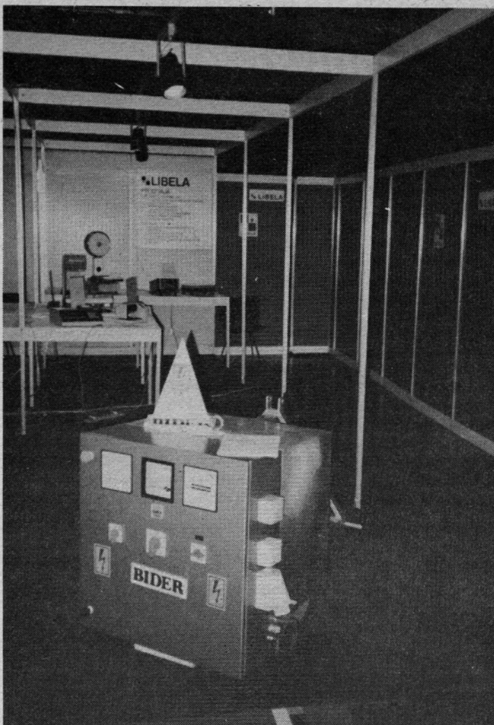
Elektroagregat na traktorski pogon BIDER. Tehnični podatki 3X220 — 380 V, 12 KW.
