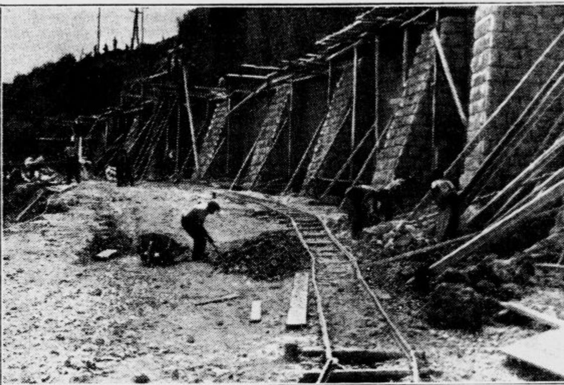
Vezava stebrišč s kamenitimi oboki (Foto Jug)
