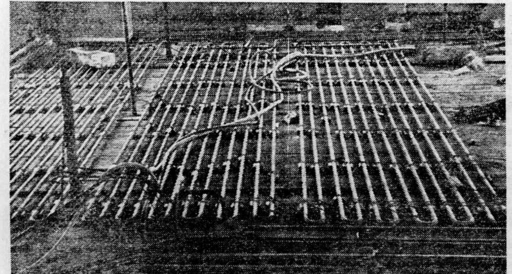
Polaganje cevi za žarilno kurjavo v stavbi MLO v Kidričevi ulici
