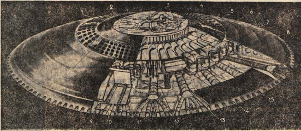
1. Pilotovo ležišče, 2. proti pritisku zavarovana pilotova kabina; 3. raketni vizir, 4. naprava za pilotiranje, 5. odprtine za dotok zraka, 6. zračne lopate, 7. zračni kompresor, 8. celice za zgorevanje plina, 9. kante za gorivo, 10. zaklopke, naprava za pilotiranje, 11. odprtini za izpuhtevanje plinov, 12. vrteča se naprava za raketne izstrelke, 13. glavni vod za eksplozivni tok, 14. turbine, 15. plinski kompresor
