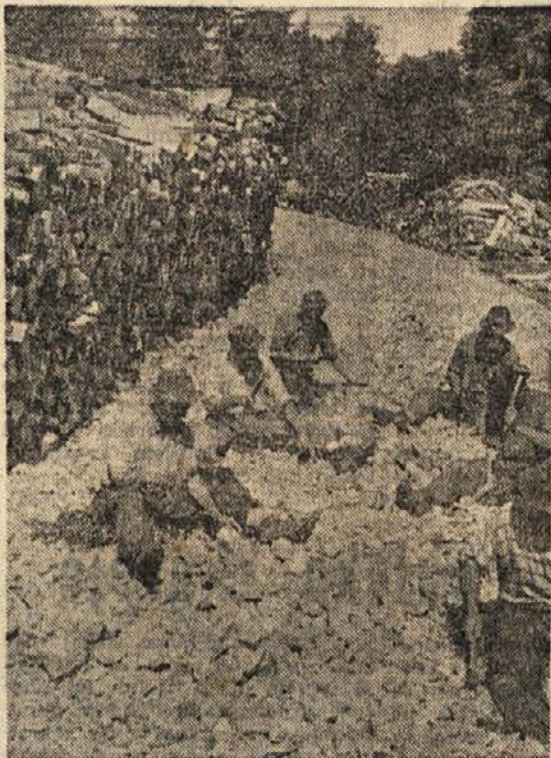
Gozdna uprava Predmeja: Toičenje gramoza na dokončani ka- mionski cesti v revirju Caven
