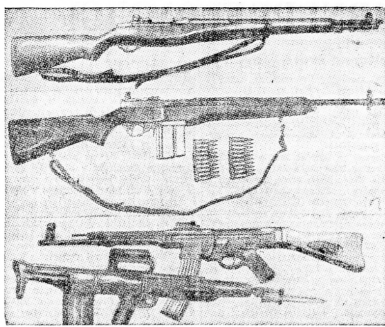
Od zgoraj navzdol: ameriška polavtomatska puška tipa Garand, dolga 1089 mm; nova ameriška puška tipa T-47, dolga 1089 mm; nemška ročna streljica za naskok MP 44, dolga 939 mm (naši partizani so ji pravili 'sesesovski šmajser'); in nova angleška puška za pchoto, tipa '0.230', dolga 990 mm.
