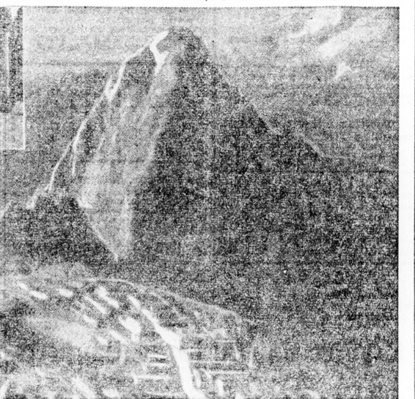
Zadnji Inki so pomrli ob koncu 17. stoletja v izgubljenem mestu Macchu-Piccu, ki je ležalo v višini 2600 metrov, zaprto od vseh strani z visokimi gorami (glej sliko).
