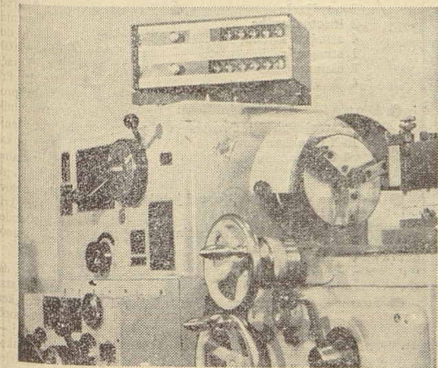
Elektronska naprava za merjenje pozicije NP na obdelovalnem stroju
