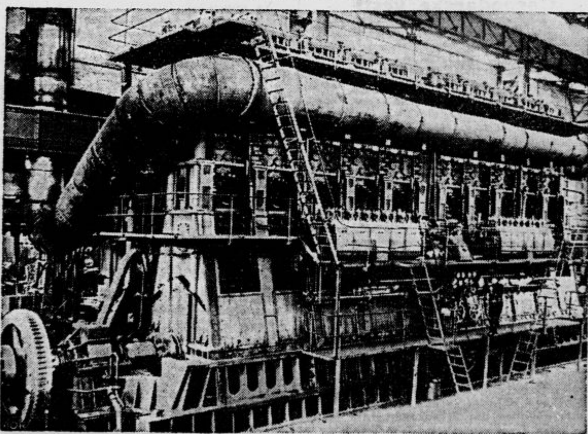
je Dieslov motor, ki so ga izdelali v Italiji in namenili za »Vulcanio«. Stroj razvija 18.000 k. s. in je največji svoje vrste na svetu
