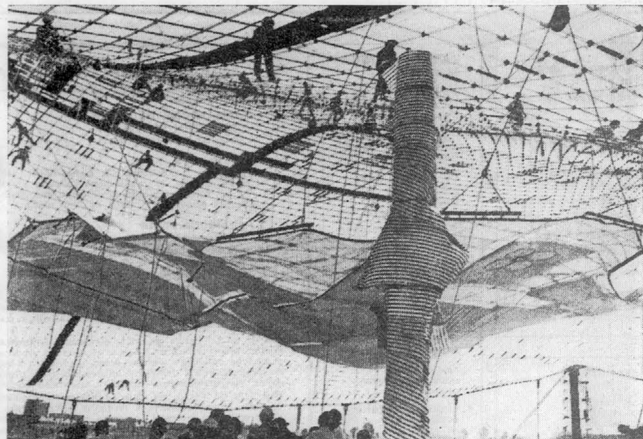
STREHA NAD OLIMPIJSKIM BAZENOM — Te dni gradijo nad dvorano za vodne športe v Münchnu ogrodje za streho, ki bo tekmovalce in gledalce na olimpijskih igrah 1972 varovala pred vročino in dežjem. Soturni podobna streha ima površino 11.900 kvadratnih metrov, v ogrodje bodo vdelali prozorne akrilne plošče. Enako streho bodo kasneje zgradili tudi nad športno dvorano in nad obema športnima igriščema. Vsa olimpijska igrišča s tribunami naj bi bila pod streho do letošnje zime. Telefot: UPI
