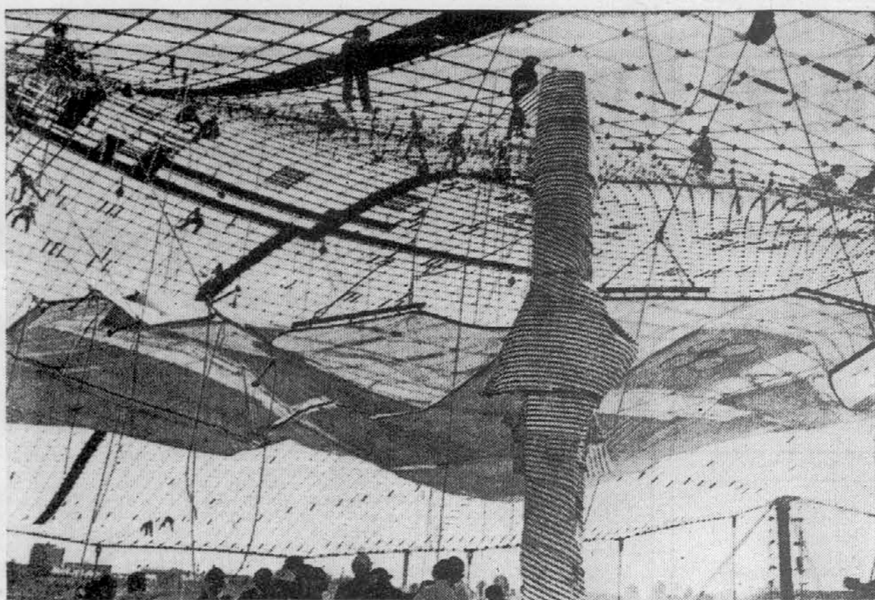
STREHA NAD OLIMPIJSKIM BAZENOM — Te dni gradijo nad dvorano za vodne športe v Münchnu ogrado za streho, ki bo tekmovalce in gledalce na olimpijskih igrah 1972 varovala pred vročino in dežjem. Soturo podobna streha ima površino 11.900 kvadratnih metrov, v ogradi bodo vdelali prozorne akrilne plošče. Enako streho bodo kasneje zgradili tudi nad športno dvorano in nad obema športnima igriščema. Vsa olimpijska igrišča s tribunami naj bi bila pod streho do letošnje zime. Telefoto: UPI
