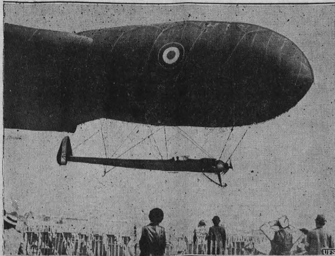
V Franciji so začeli graditi novovrstne opazovalne zrakoplove, katere vodi letalni propeler, kakor je videti na sliki. Te vrste zrakoplovi se veliko bolj hitro in lažje kretajo, kakor drugi tipi.
