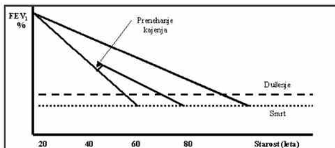
Slika2: Upad FEV1 s staranjem pri zdravem nekadilcu in pri bolniku s KOPB. Za časa življenja normalen upad FEV1 ne povzroči težav z dihanjem. Pri bolniku s KOPB je upad hiter. Posledica so vse večje težave z dihanjem in končno smrt. Če bolnik preneha kaditi, doseže normalen upad FEV1.
