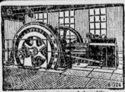
LANZOVE vročeparne Lokomobile s naravnost vezano Dynamo.
