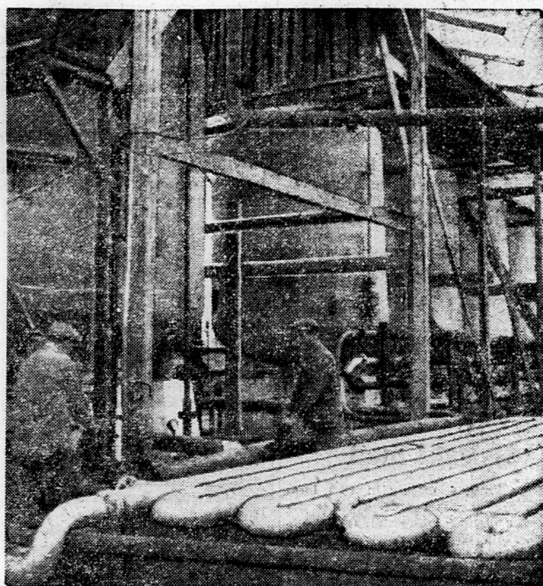
Pionirji naše industrije narite v Dolnji Lendavi so pred dvema letoma zgradili brez vsake tuje pomoči prvo poskusno napravo degazolizno, v kateri iz zemeljskega plina izločajo gorivo, ki je važen sestavni del letalskega bencina. Po prvih uspehih se je pridobivanje gorilna, butana in propana iz zemeljskega plina hitro razvilo. Za zajemanje in predelavo zemeljskega plina bodo letos zgradili naprave v vrednosti 200 milijonov din. Med drugim grade prvo visokotlačno degazolizno. Slika nam kaže del sedanjih naprav za pridobivanje gorilna.
