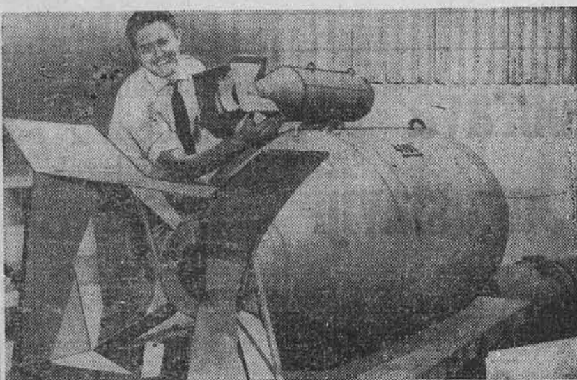
Slika tega 4,000 funtov težkega "block busterja" je bila vzeta v Wright Field, Ohio, skupno s svojo majhno sorodnico, 100 funtov težko uničevalno bombo. Prva bomba je slučajno danes največja bomba, ki jo rabijo Zedinjene države, toda britske bombe tehtajo 8,000 funtov.
