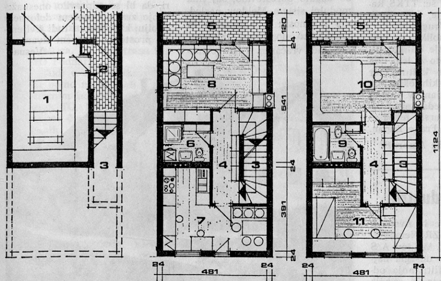
KLET PRITLIČJE ETAŽA VRSTNA HIŠA IZO VH 6 b — VARIANTA I: 1. Garaža, 2. Vetrolov, 3. Stopnišče, 4. Hodnik, 5. Loža, 6. WC, tuš, 7. Kuhinja, jedilni kot, 8. Dnevna soba, 9. Kopalnica, 10. Spalnica, 11. Soba
