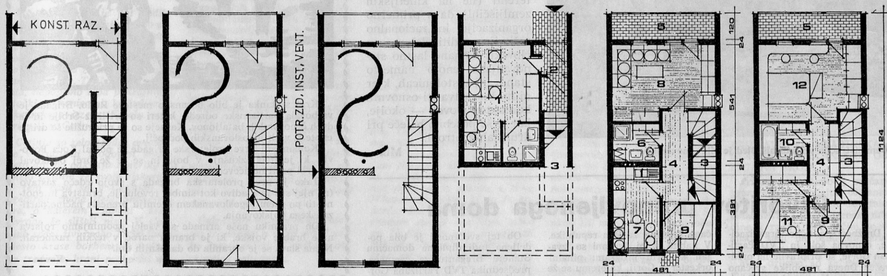
KLET PRITLIČJE ETAŽA VRSTNA HIŠA IZO VH 9 b — VARIANTA II: 1. Garsonjera, 2. Vetrolov, 3. Stopnišče, 4. Hodnik, 5. Loža, 6. WC, tuš, 7. Kuhinja, jedilni kot, 8. Dnevna soba, 9. Kabinet, 10. Kopalnica, 11. Soba, 12. Spalnica
