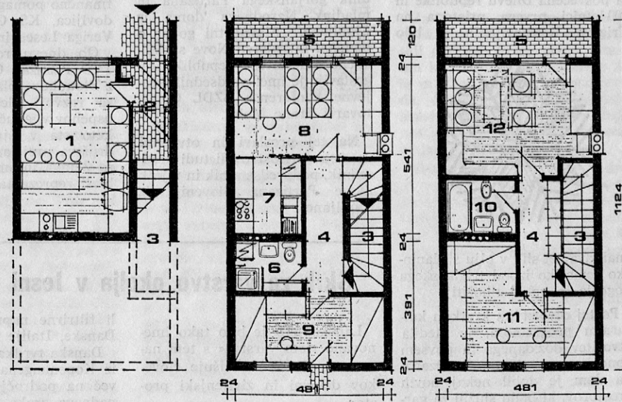
KLET PRITLIČJE ETAŽA VRSTNA HIŠA IZO VH 9 b — VARIANTA III: 1. Posebna soba, 2. Vetrolov, 3. Stopnišče, 4. Hodnik, 5. Loža, 6. WC, tuš, 7. Kuhinjska niša, 8. Jedilni kot v dnevni sobi, 9. Soba, 10. Sanitarije, 11. Soba, 12. Spalnica dnevna soba
