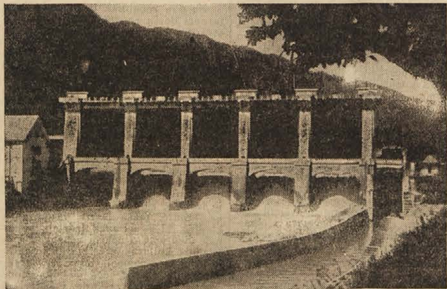
Zajezni most elektrarne Fale s glavnimi zapornicami
