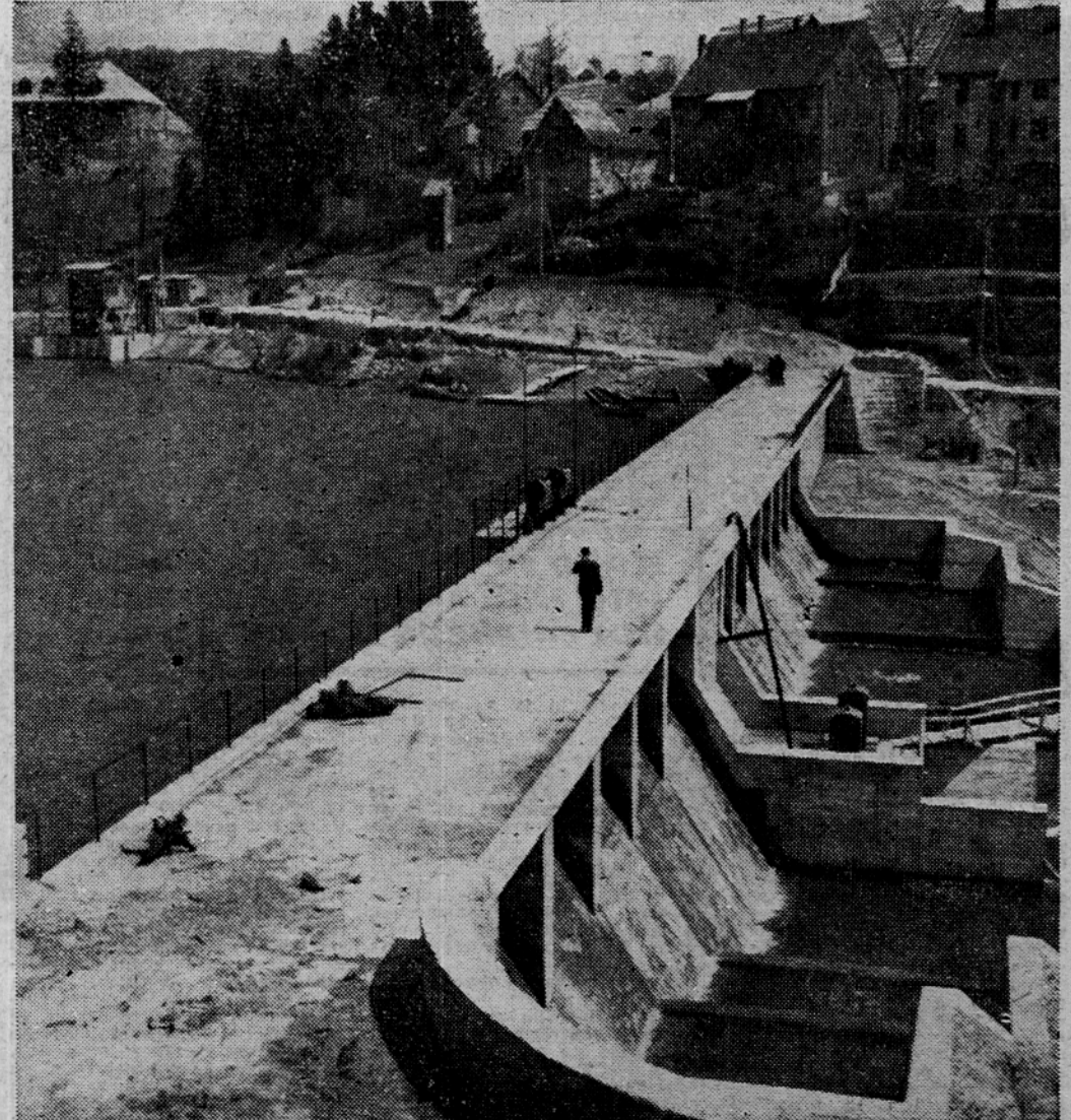
Cez pregrado umetnega jezera Bajer so speljali cesto do Fužin. Ob jezeru (na levi strani slike) je majhna hišica za avtomatične čistilne naprave. S tega mesta odteka voda po 10 km dolgi poti skozi predor pod Fužinami, cevovod Ličko polje, predor Koblijak-Razomir in Jekleni tlačni cevovod do 650 metrov niže ležeče podzemeljske strojnice v Triblju nad Crikvenico.
