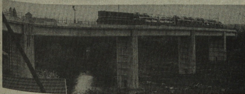
Prvi vlak je iz tovarne IMV odpeljal 25. aprila. Most so zgradili delavci TOZD GE nizkih gradenj iz Maribora
