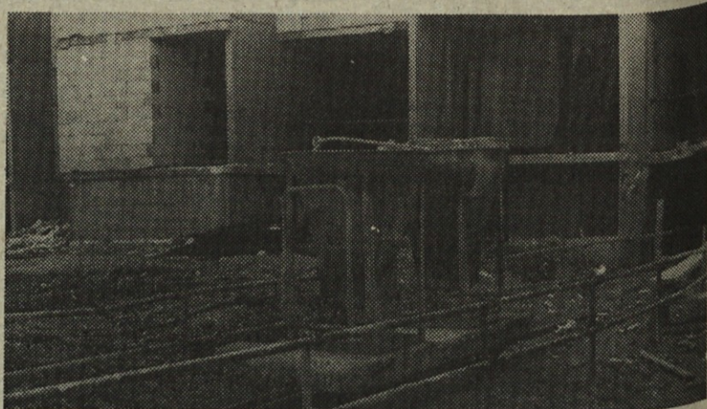
Na koncu tira sta kadunji v dosegu obeh žerjavov, ki pokrivata delovno območje vseh štirih objektov podkvice C
