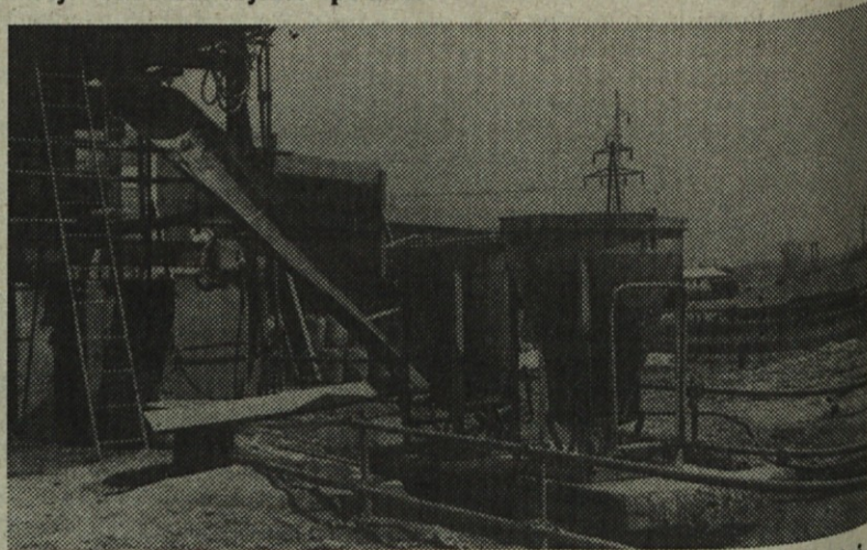
Kadunji za beton se polnita po železnem žlebu, ki je v naklonu 36 stopinj
