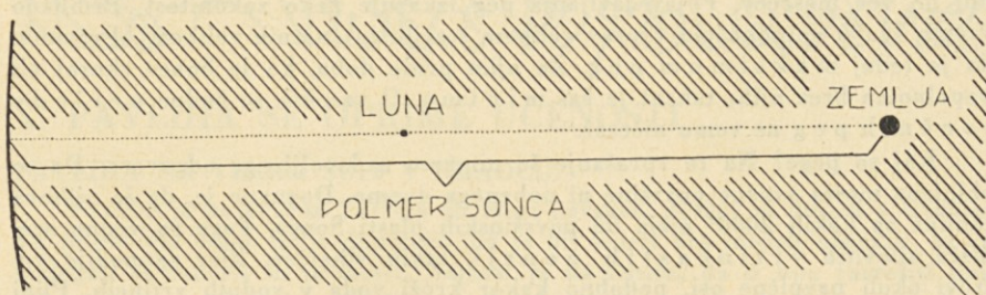
Zemlja, luna ter njuna razdalja v primeri s soncem.
