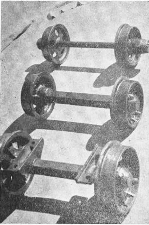
Ravenski kolesni stavki za rudniške in gradbene vagonete.
