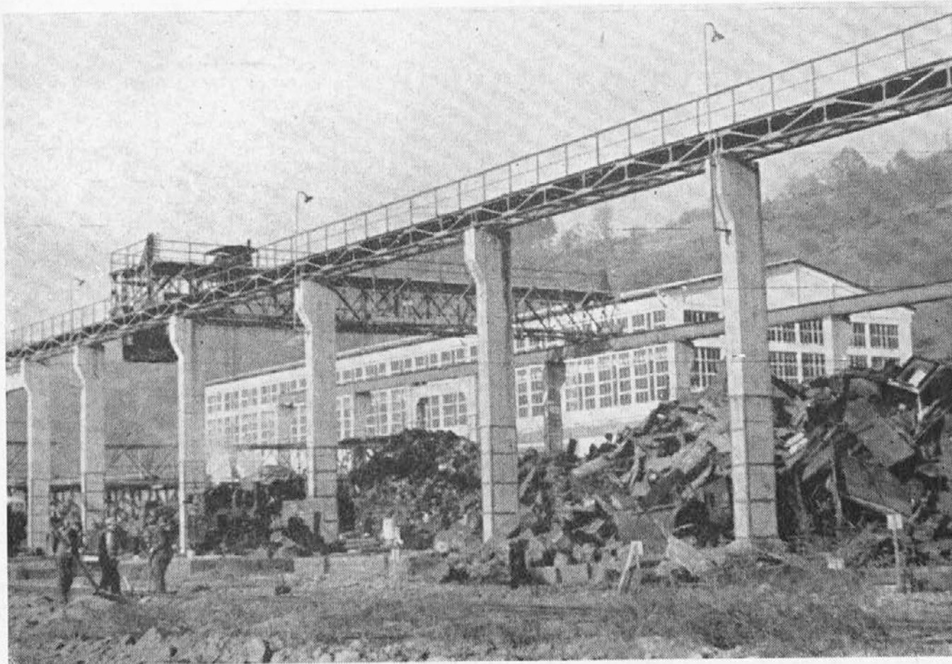
Tu vidimo na isti sliki začetek in konec tovarne: V ospredju del skladišča starega železa na dohodu, zadaj pa novo odpremno skladišče železarnice.
