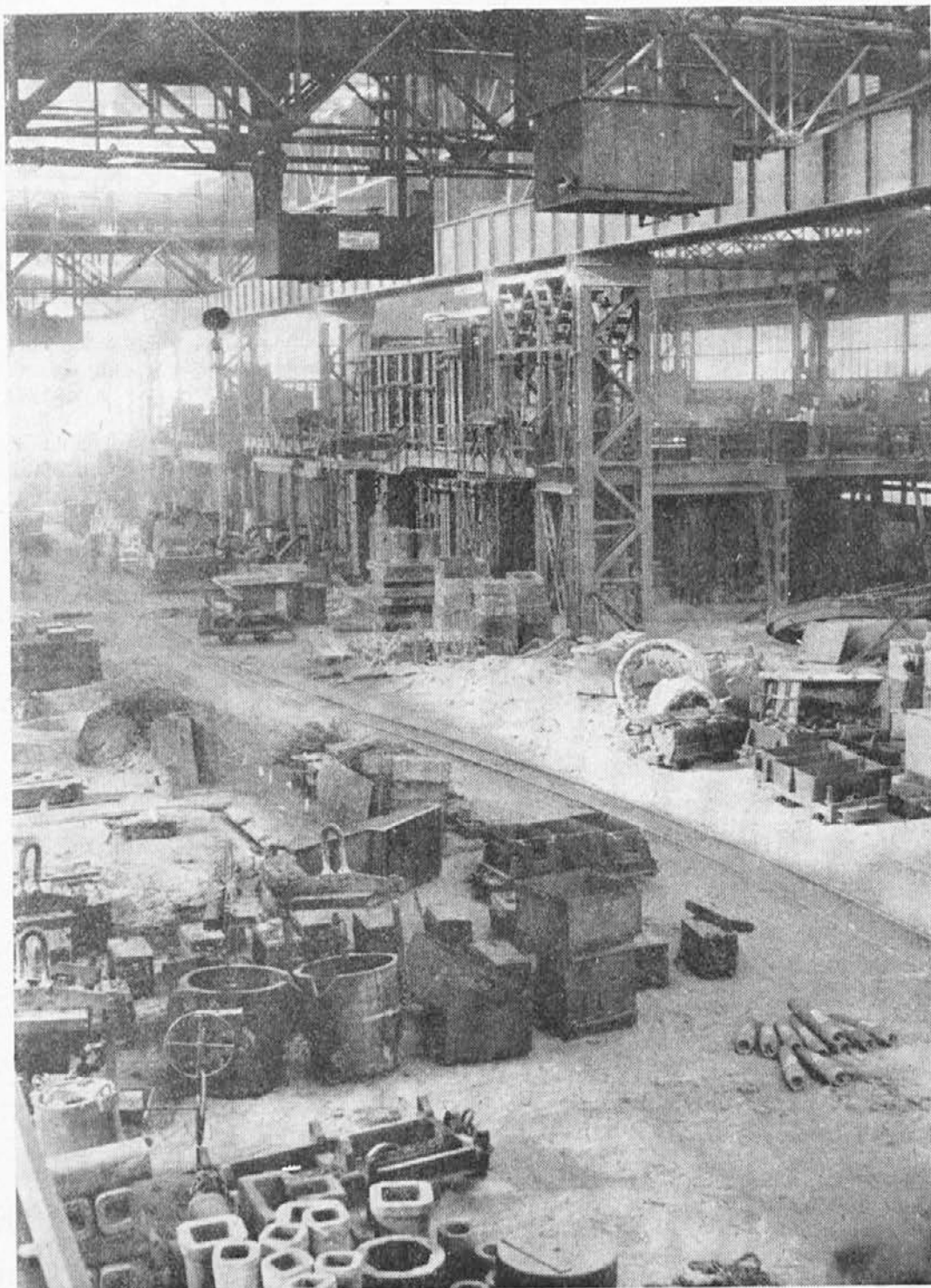
V jeklarni.
