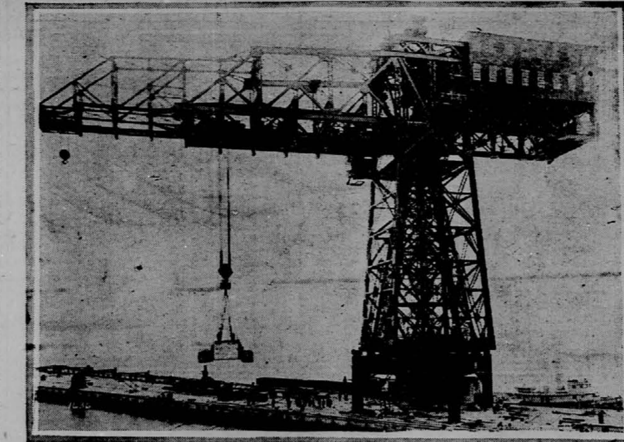
NAJVEČJA DVIGAČA NA SVETU. Zgrajena je bila za ameriško mornarico. Nacun funtov 245 čevljev visoko. Zgradili so jo v Philadelphiji.
