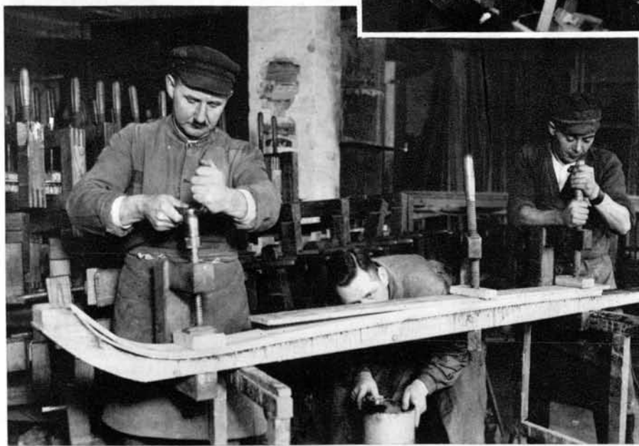
Oblanje smučk s posebnim električnim obličem.
