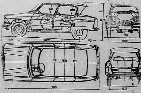
Glavne dimenzije novega »AMI 6«.
