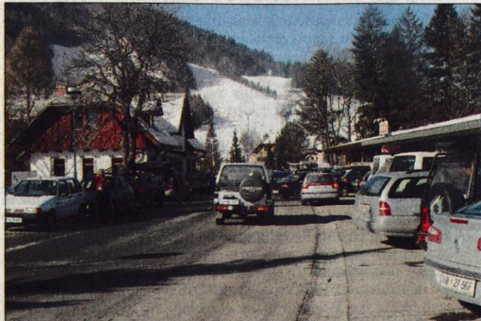
Vožnja skozi vas je pravi podvig.
