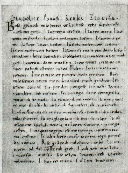
Brižinski spomeniki, praslovenski rokopis iz 10. stoletja.
