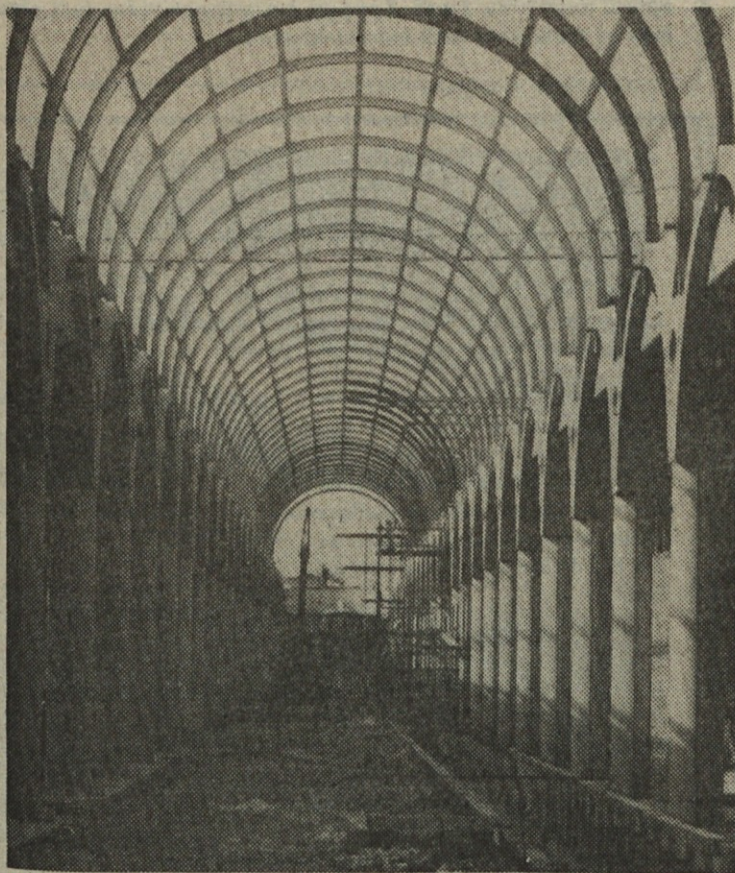
Osrednji del mariborske avtobusne postaje bo po dograditvi podoben pokriti ulici.
