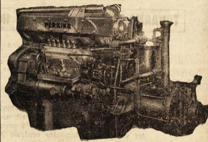
Tipa „56-M“ specialni ladijski motor
