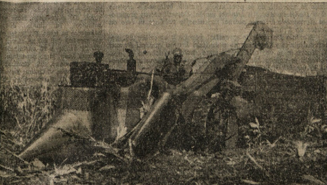
Enovrstni stroj za obiranje koruze, kot ga uporabljajo na ameriških farmah; s kljunom odkljuje koruzna stebelja do stranskih žlebov, kjer jih posebni noži odrežejo, notranji mehanizem pa potrga storže od stebel
