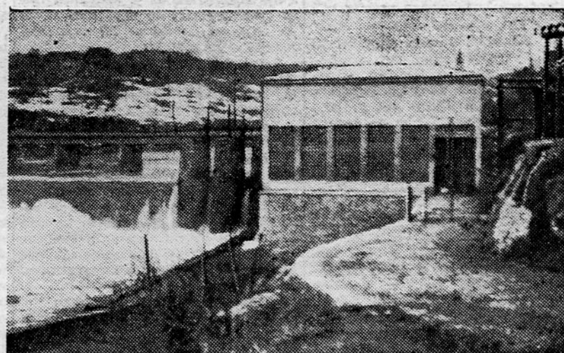
Nova hidrocentrala Ozalj II. na Kolpi bo začela danes redno obratovati z obema agregatoma in skupnim učinkom 2200 kilovatov. Naprave nove elek. trarne so izdelali v Litostroju in v tovarni Rade Končar; montažna dela pa so opravili delavci Hidromontaže iz Maribora. Slika nam kaže strojno novo centrale in del pregrade, ki služi tudi stari centrali ob levem bregu Kolpe.
