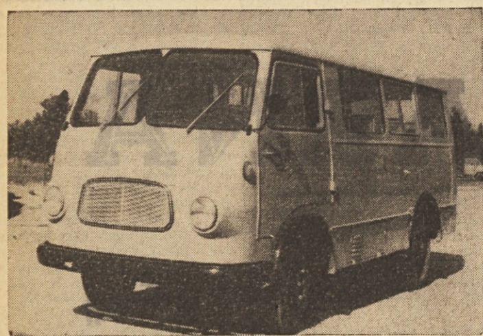
Kombi-bus »TAM 2000 CB«, 12 sedežev Diesel motor 55 KS - nov proizvod TAM
