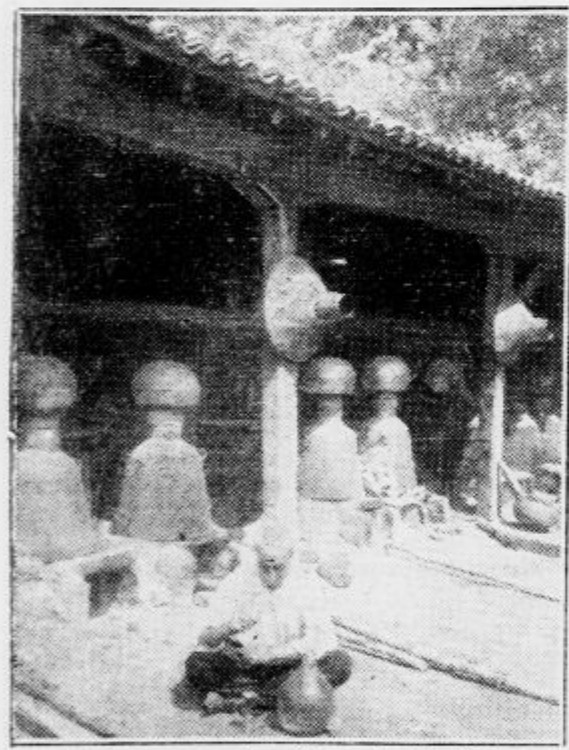
Preprosta »kmečka« distilacija
