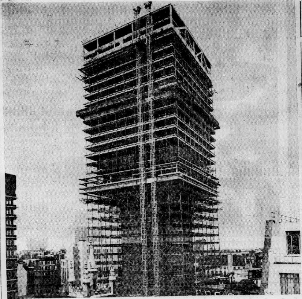
GRADITEV OD ZGORAJ NAVZDOL — Poslovni nebotičnik (30 nadstropij) za neko zavarovalnico gradijo v Londonu po sistemu »dežnik«. Najprej so postavili osrednji del, nato pa so začeli dograjevati pisarniške prostore od zgoraj navzdol. Stamba je visoka 118 m, kvadratni floris ima stranico 37,8 m, v osrednjem delu je 12 hitrih dvigal, zraven njih so stopnišča in umivalnice. Vsi poslovni prostori s skupno površino skoraj 28.000 kvadratnih metrov imajo klimatične naprave.
