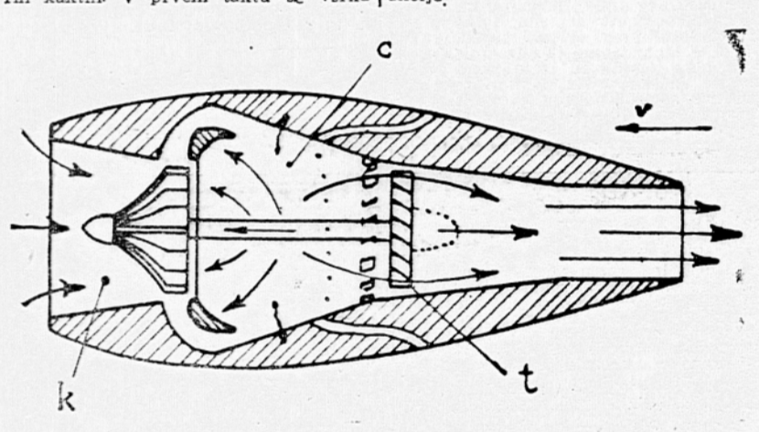
Shematični prikaz reaktivnega motorja na puh v prerezu
