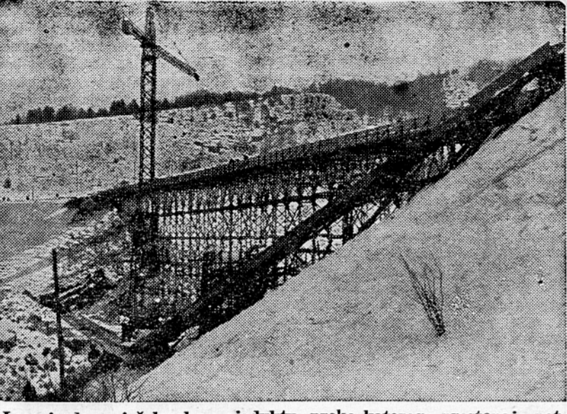
Leseni oder pri žalenskem viaduktu, preko katerega prestopajo potniki. V ospredju tik ob odru je dograjen opor za betoniranje viaduktnega opornika
