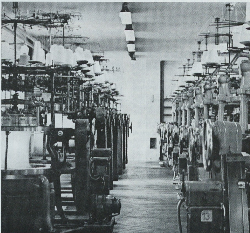
Okrogli pletilni stroji, na katerih nastajajo BETI pletenine
