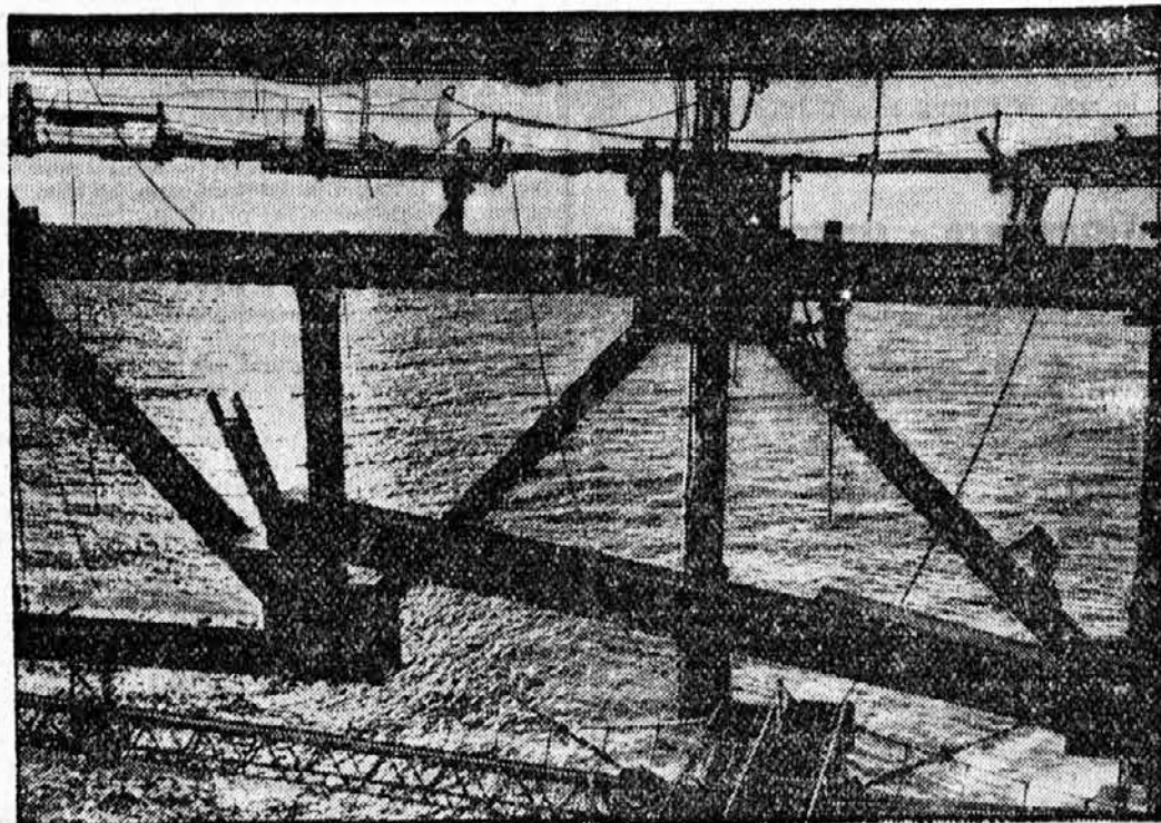
Pri graditvi večjih mostov čez nevarne reke potegnejo široko mrežo, da ne bi kak delavec padel v vodo.
