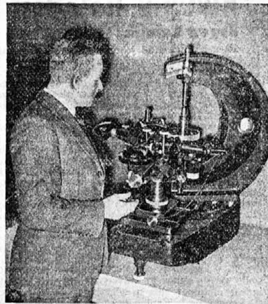
V Nemčiji so izumili tole pripravo, s pomočjo katere preizkušajo pravilnost zobčastih koles.
