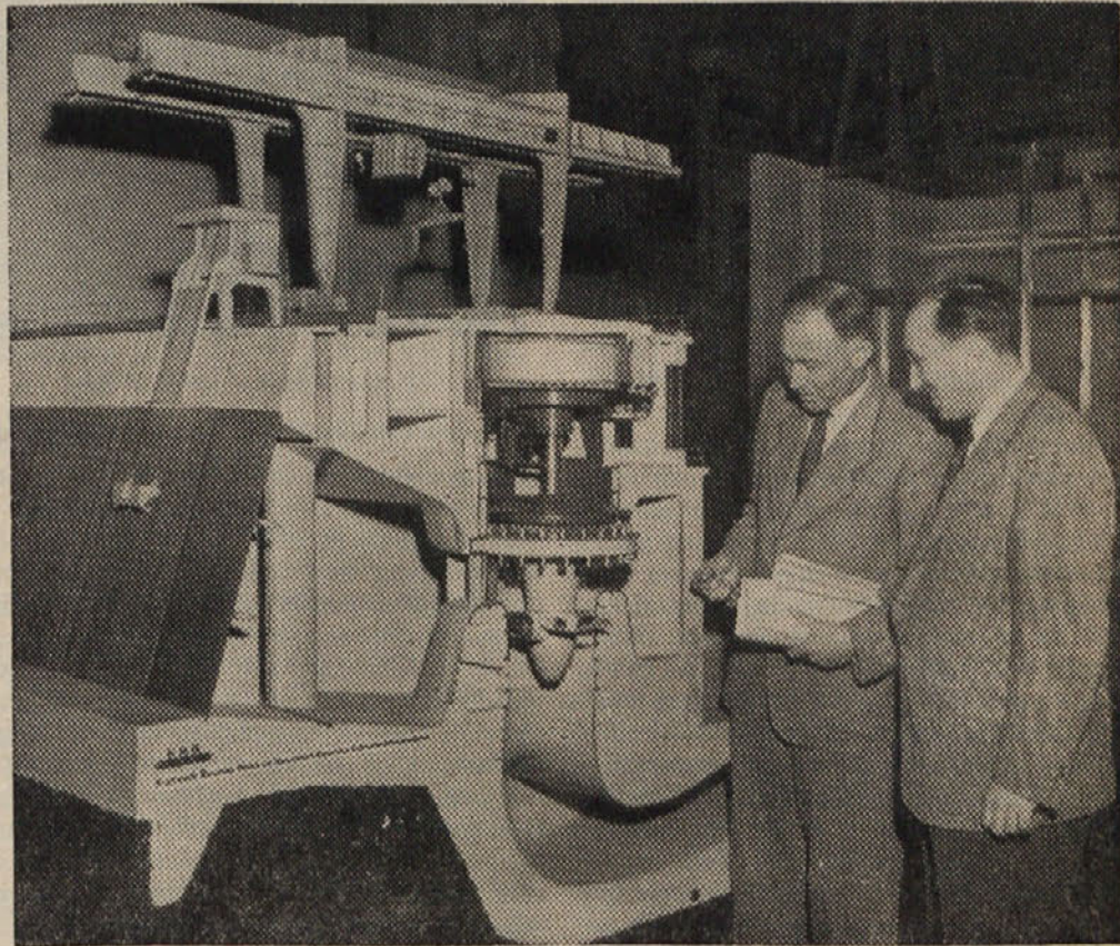
Na Dunaju je bila razstava o pridobivanju električnega toka. Te model, ki ga vidimo na sliki, je iz elektrarne na avstrijsko-bavarski meji Simbach-Braunau. Slika kaže prerez skozi turbino in generator.
