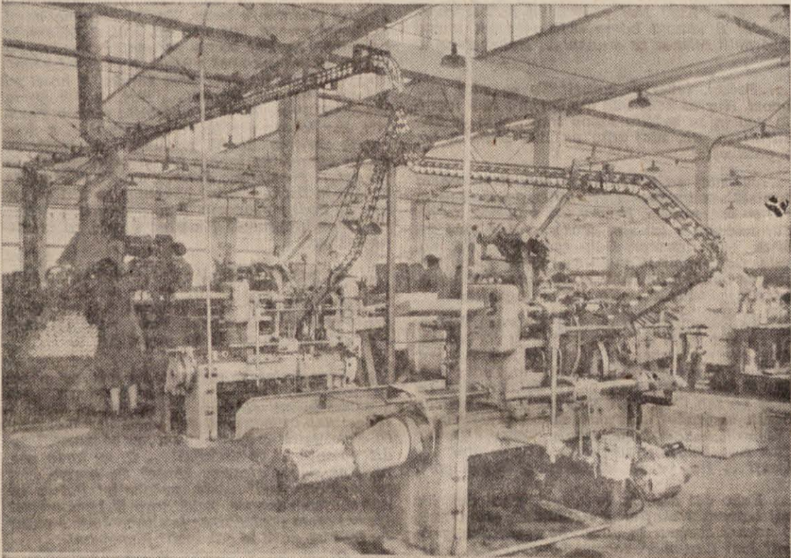
Avtomatska proizvodnja konzervnih skatel.
