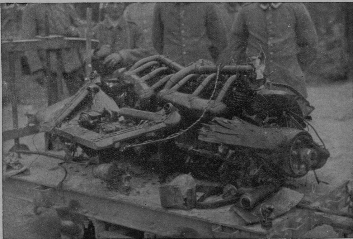
Ostanki motorja, sestreljenega in uničenega sovražnega letala za francosko fronto.
