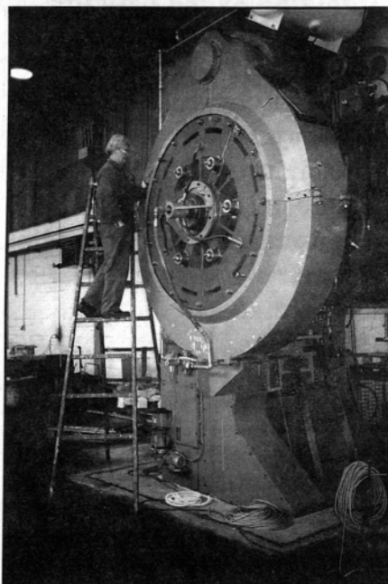
Končna montaža 1.500-tonske stiskalnice (foto: Savinjščan)
