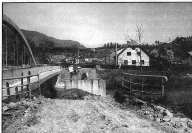
Starega mostu preko Savinje ni več (foto: Ciril Sem)
