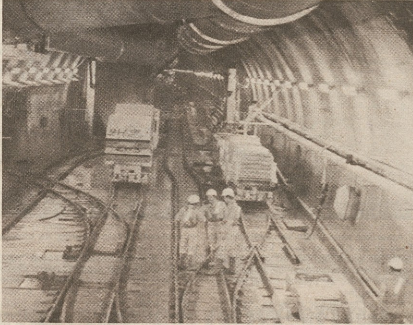
Predor, ki bo povezoval Francijo z Veliko Britanijo, zadobiva konkretnije oblike. Francoski delavci so že »zgradili« 3699 metrov dolgo galerijo pod Rokavskim prelivom, britanski in francoski bagerji pa bi se morali srečati leta 1990, tri leta pred predvidenim odprtjem evrotunela (Telefoto AP)
