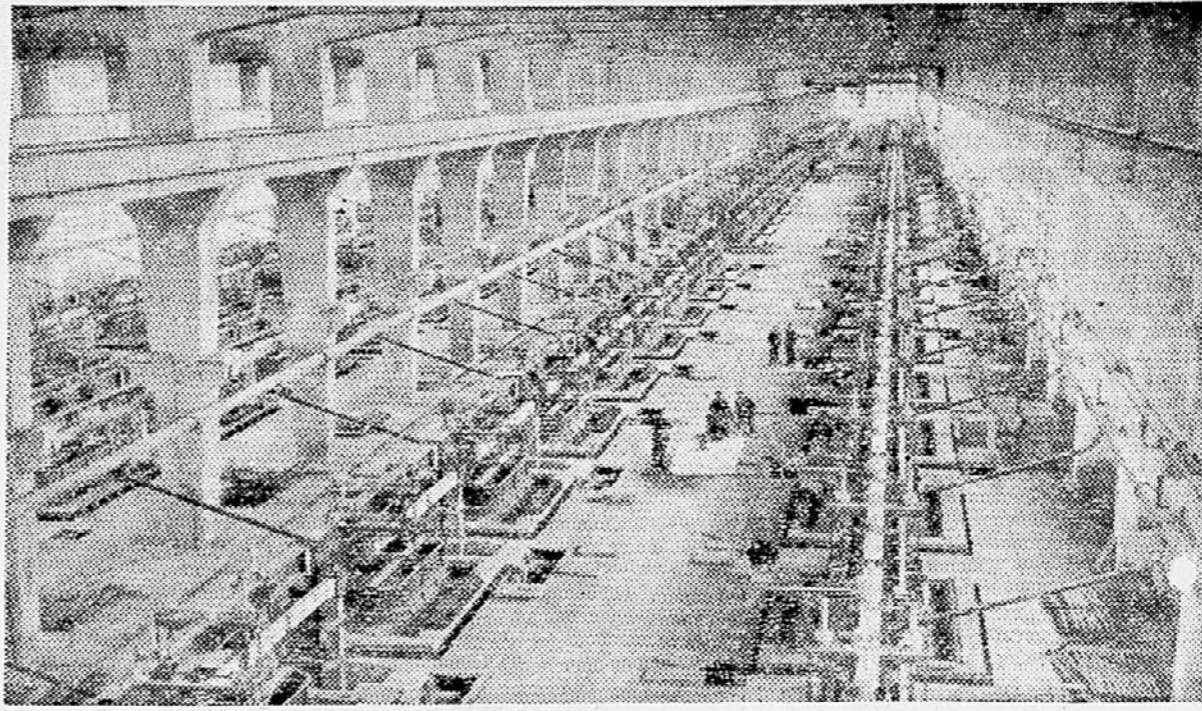
Notranjost ene izmed hal v tovarni aluminija v Kidričevem
