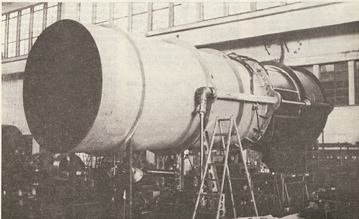
Zapiralo Howell-Bunger za Hemren Dam v montaži
