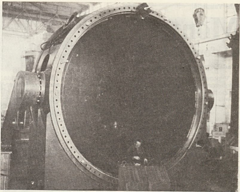
Loputa premera 5000 mm za Hemren Dam je v fazi poizkusne montaže (Foto: J. Žlebnik)
