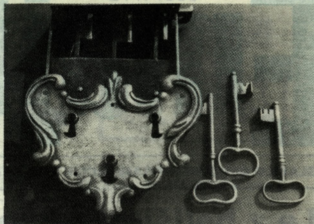
Ključavnica za skrinje, omare in blagajne iz 18. stoletja. Kleščni mehanizem s tremi zapahi. Vsak zapah se je zaklepal posebej, odtod 3 ključi. Cehovsko blagajno so lahko odprli samo ob navzočnosti vseh treh vodilnih cehovskih članov.
