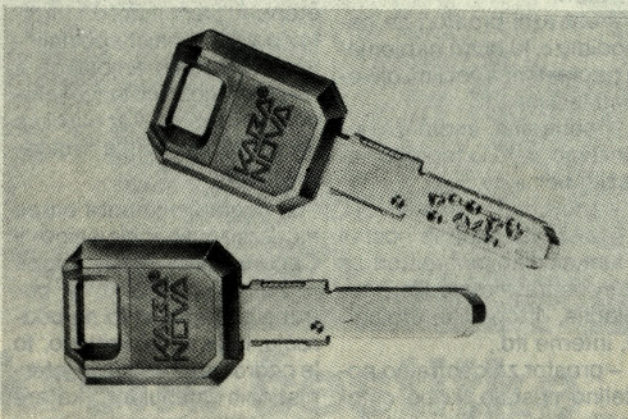
Ključi za magnetno-elektronsko ključavnico. Na stebelu ključev so magnetki, mikroelektronika je vgrajena v glavo ključa.
