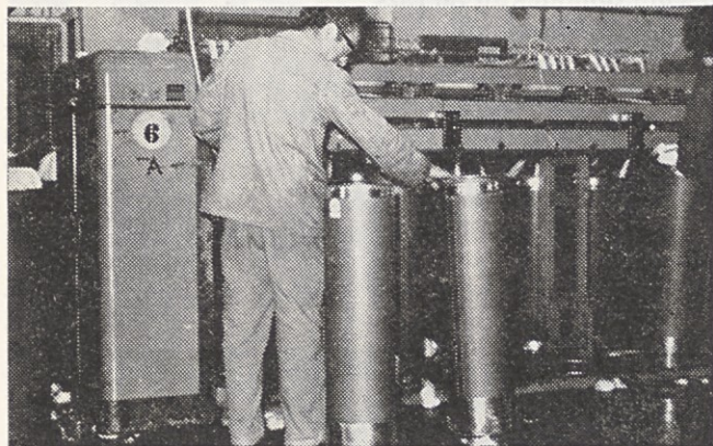
Raztezalko Ingolstadt smo uredili tako, da se pramen lahko uporablja kot predpreja na brezvretenskem stroju BD-200 RC.
