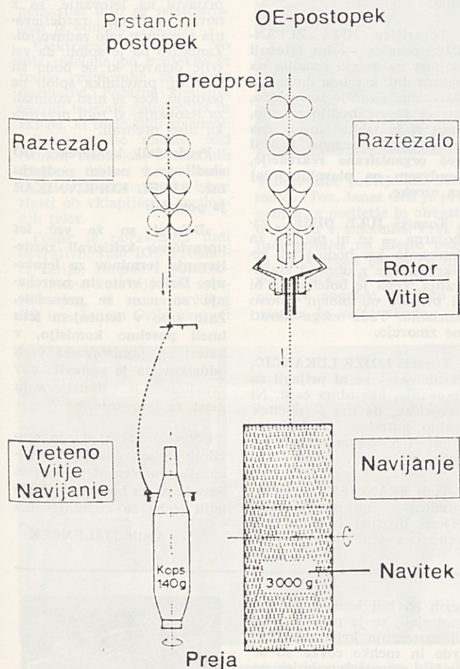
Primerjava konvencionalnega prstančevega postopka in predilnega postopka OE z rotorjem odnosno predilno turbino.
