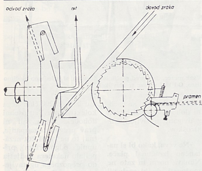
Shema predilne naprave
