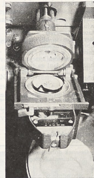
Odprto predilno telo. Vidi se predilna turbina in separator.
