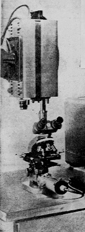
Predvsem šolam in drugim vzgojnim ustanovam je namenjena kombinacija mikroskopa in televizorja, izdelek tovarne optičnih predmetov v Rochesteru. Učenci si lahko na televizorskem zaslonu ogledajo povečano sliko snovi pod mikroskopom
