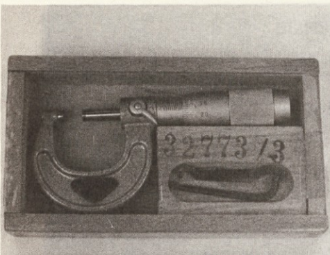
Mikrometer za posebno precizna merjenja pri polnjenju meri do stotinke milimetra natančno.
