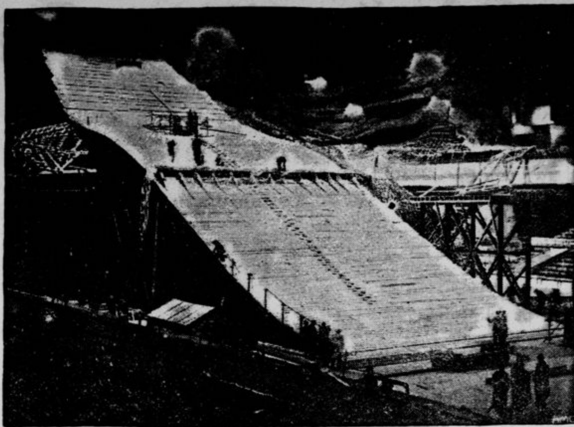
Razstavno dvorano Earl Court v Londonu so spremenili v dvorano za zimске sporte, kjer bodo smučarji lahko tekmovali v skokih. Posebne naprave bodo nametale na skakalnico v treh minutah 80 cm debelo plast snega
